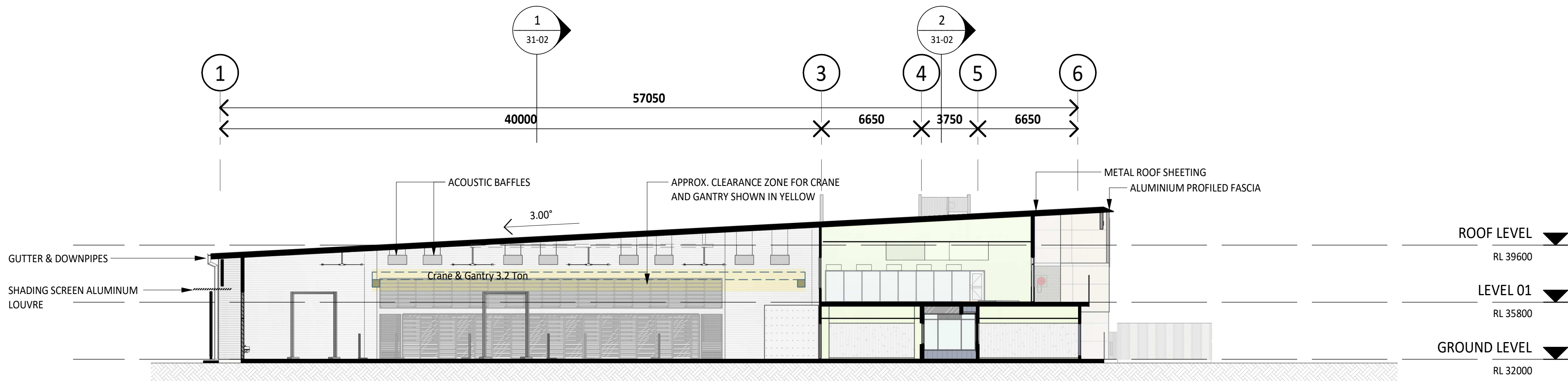
1 21-01 GA SECTION 01 1 : 200
