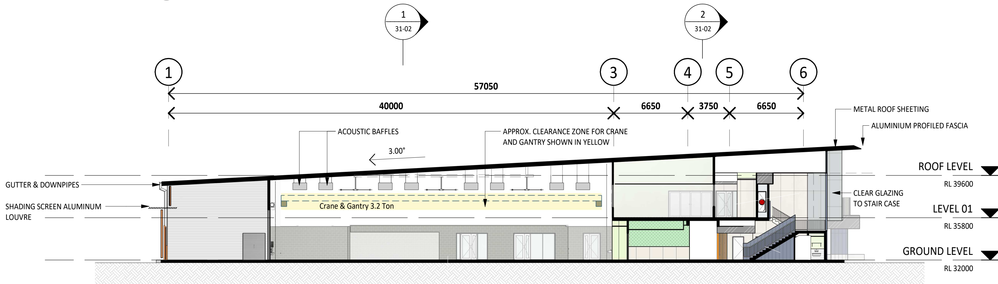
1 21-01 GA SECTION 01 1 : 200
